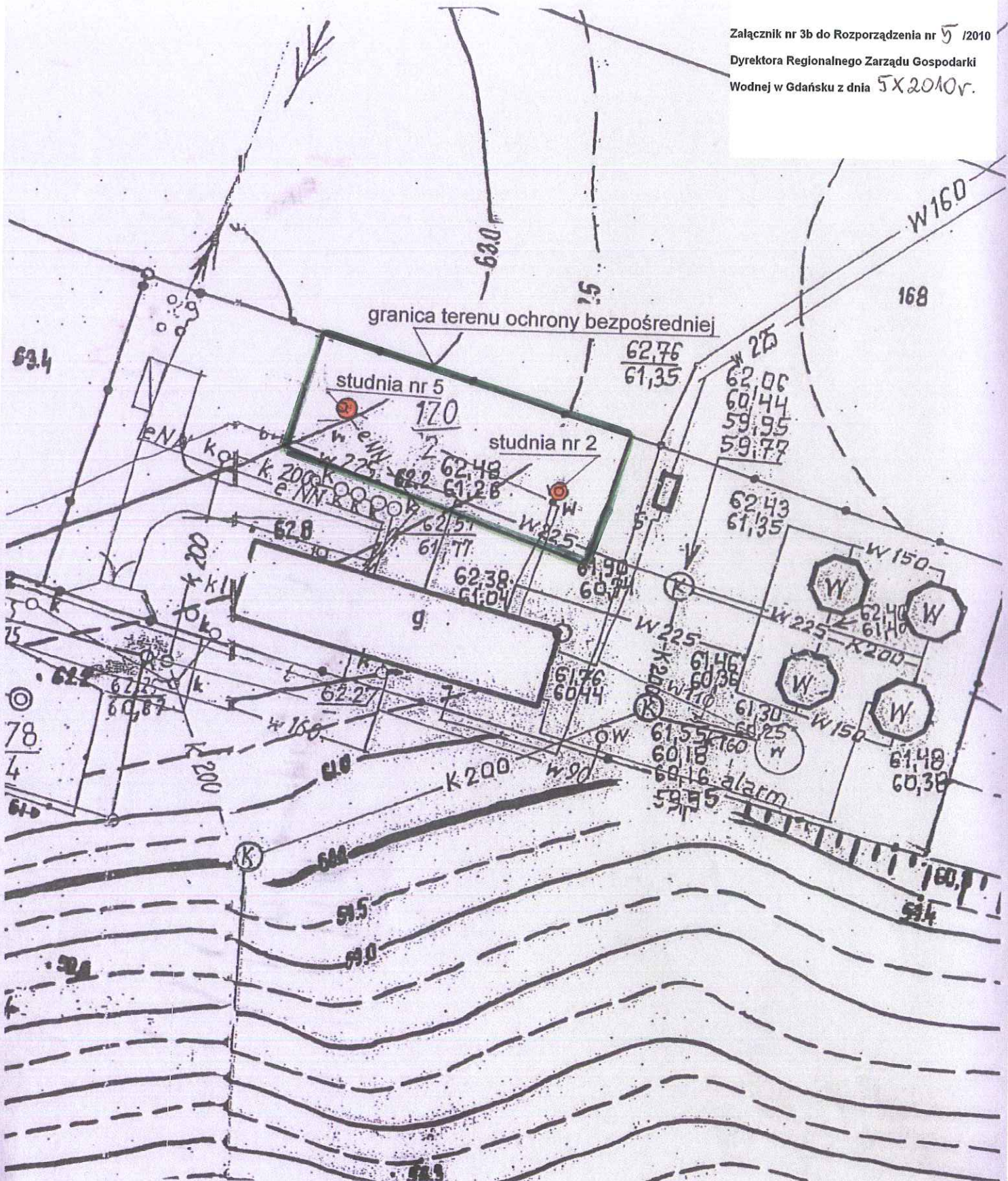
MAPA SYTUACYJNO – WYSOKOŚCIOWA terenu ochrony bezpośredniej ujęcia wody w m. Górna Grupa studnie nr 2 i nr 5 skala 1 : 500
